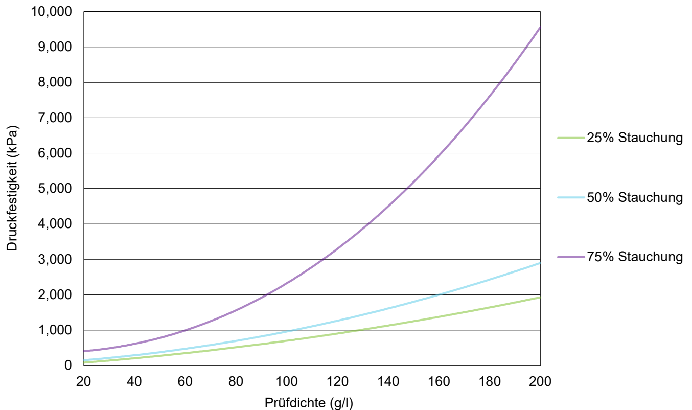
Druckfestigkeit - ISO 844
